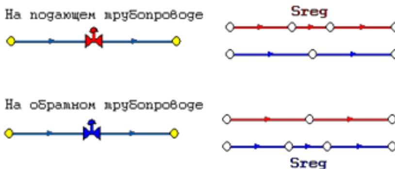
Рисунок 17 – Дросселирующие устройства
